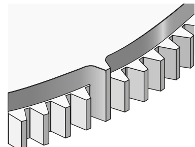
Z = Referenzmarke - Zahn Standard-Messzahnrad
