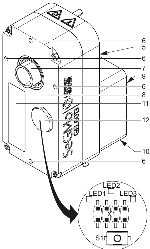
Positionierantrieb mit Durchgangshohlwelle - Rückseite
